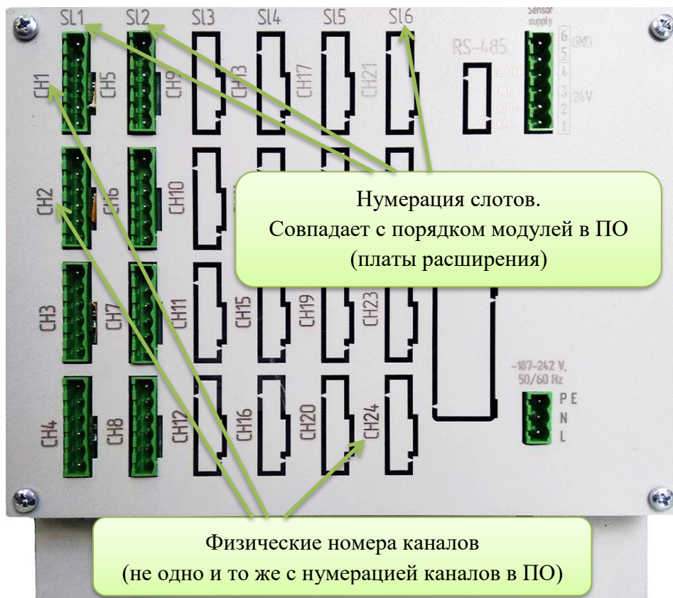
Рис.5. Обозначения на задней крышке прибора.
